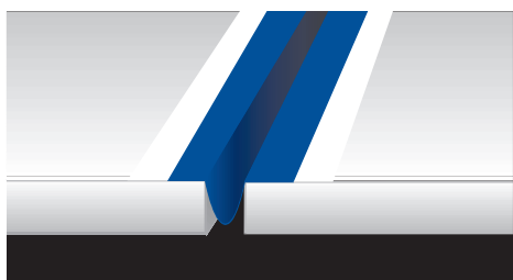
In een omega-vorm \Omega aanbrengen van Mapeband in een dilatatievoeg
